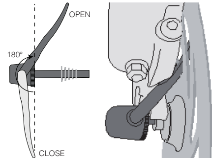
図1. 180°以上開いた状態の クイックリリースレバー
